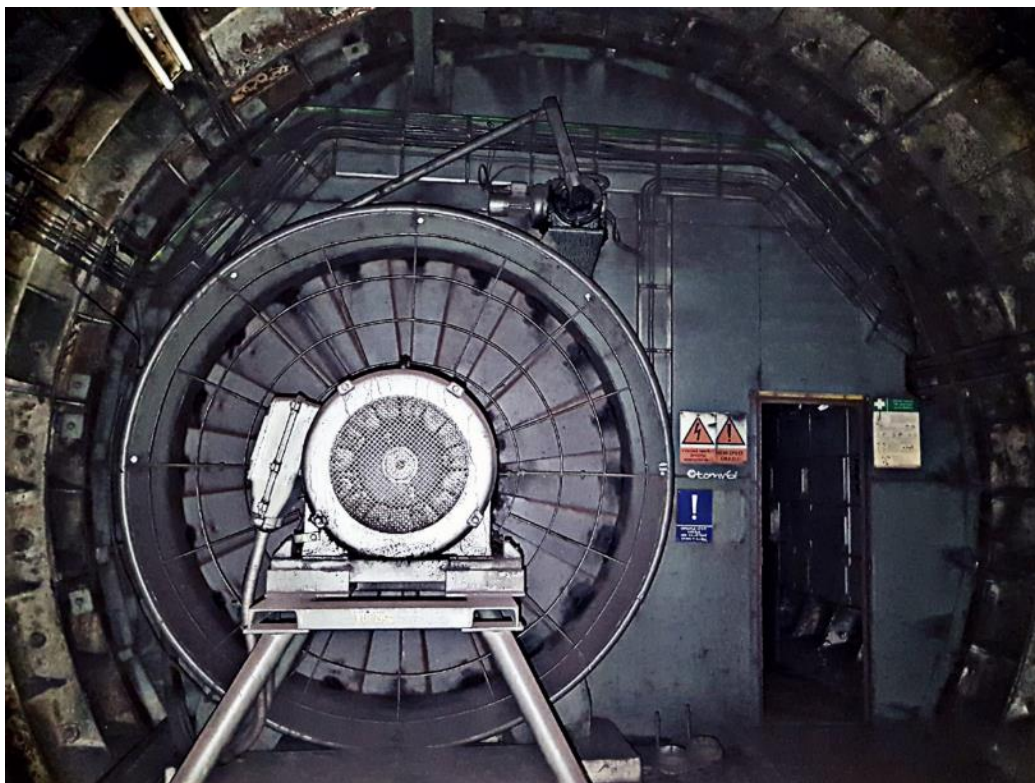
Příloha 3 – Zavřený mžikový uzávěr ventilátoru
