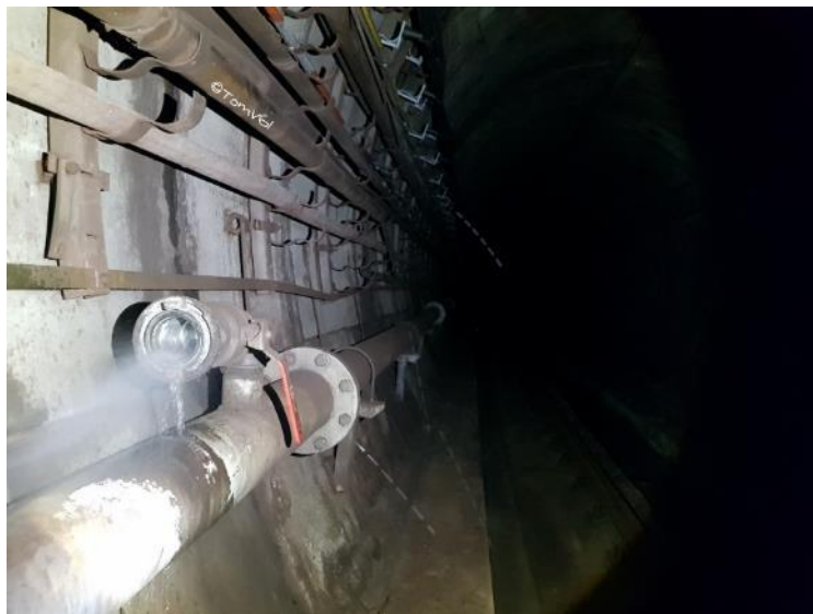
Foto 13 - Tunelový vodovod
