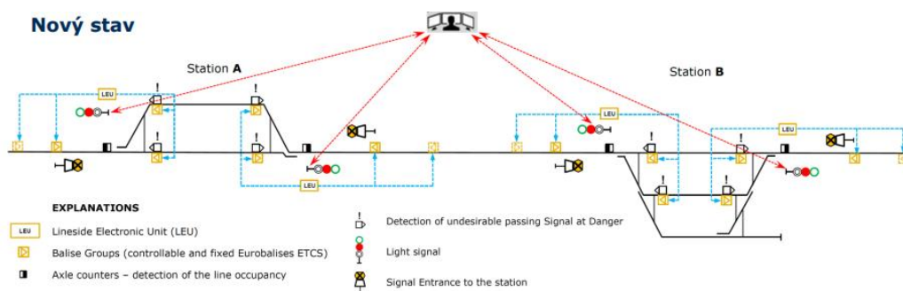
Obrázek 3: Schéma vlakového zabezpečovače ETCS Stop v dopravnách D3 3
